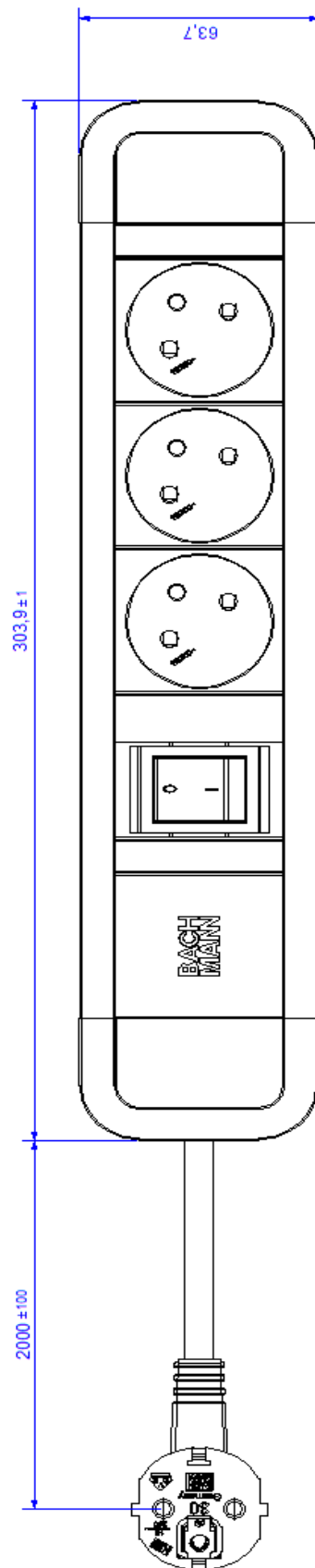
H05VV-F 3G1,5mm 2 schwarz / black mit Winkelstecker CEE 7/7 / Angled plug CEE 7/7
